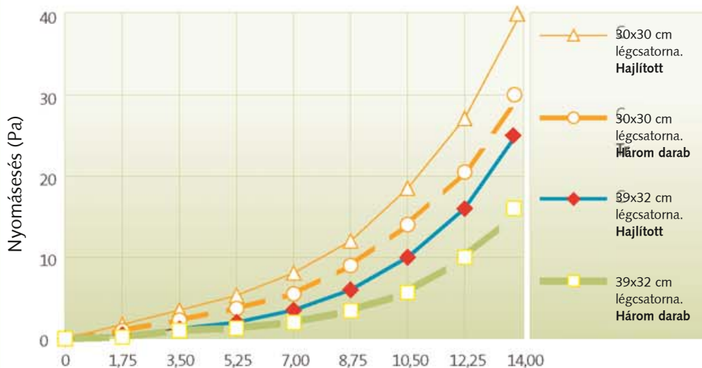
Nyomáskereső a hajlított könyök és a 3 egyenes szakaszból álló könyök idomok esetében:
